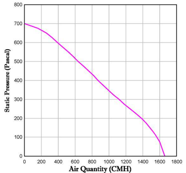
Fan Model : AF315EE
