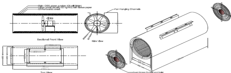
Jet Fan - 315mm dia
