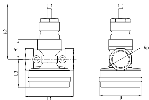
Fig 3: DN32-DN50
